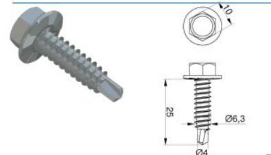
Samozávrtný šroub 6,3×25
