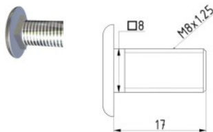
Šroub s aretací
