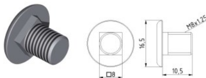
Krátký šroub do kolejnice
