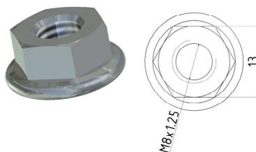
Matice s vroubkováním M8
