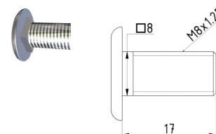
Šroub s aretací M8x17
