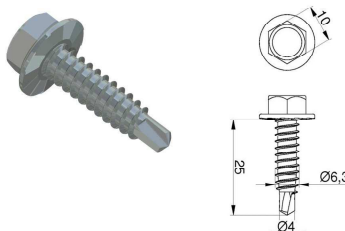
Samozávrtný šroub 6,3×25mm
